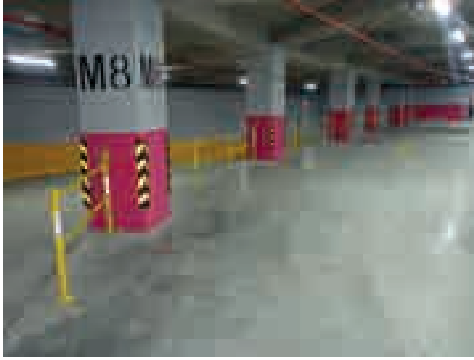
Belediye Binası Otopark Korkulukları
